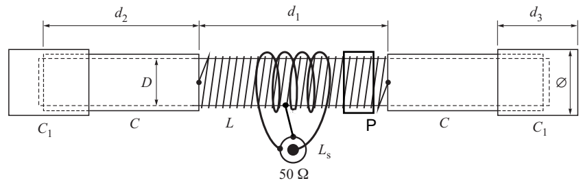
Slika 3. - Nacrt antene 9A4ZZ bipol
